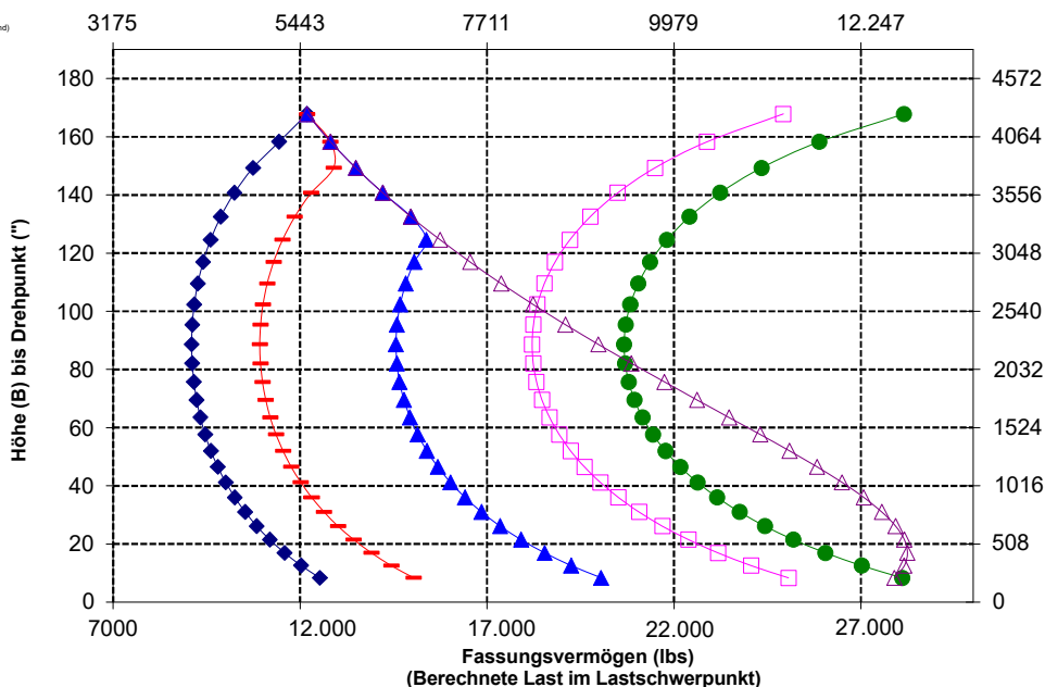
Fassungsvermögen (kg) (Berechnete Last im Lastschwerpunkt)
