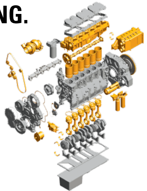
Aufbau Cat Dieselmotor
